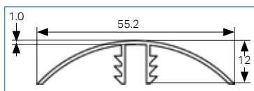
Unterseite - Freiform
